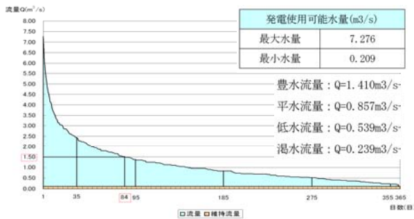
図-3 平沢川流況曲線図（5ヶ年平均）
