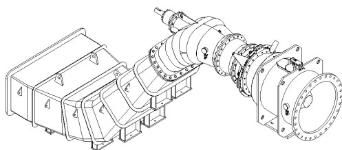
図-5 S型チューブラ水車
